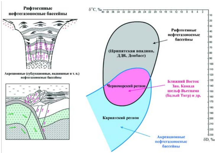
Рис. 2. а) Геодинамические типы нефтегазоносных бассейнов Украины и их изотопно-геохимические отличия.
