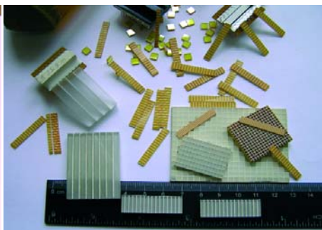
Образцы 1D-линеек и 2D-матриц, изготовленных на основе \text{ZnSe} и оксидных кристаллов
