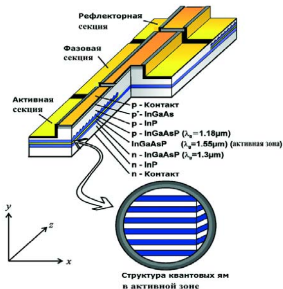
Рис. 1. Применение теории возмущений для синхронизации колебаний в оптическом лазере
