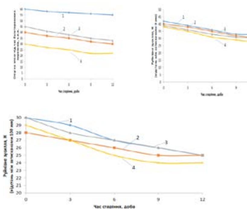
Рис. Залежність фізико-механічних показників паперу від часу штучного старіння
