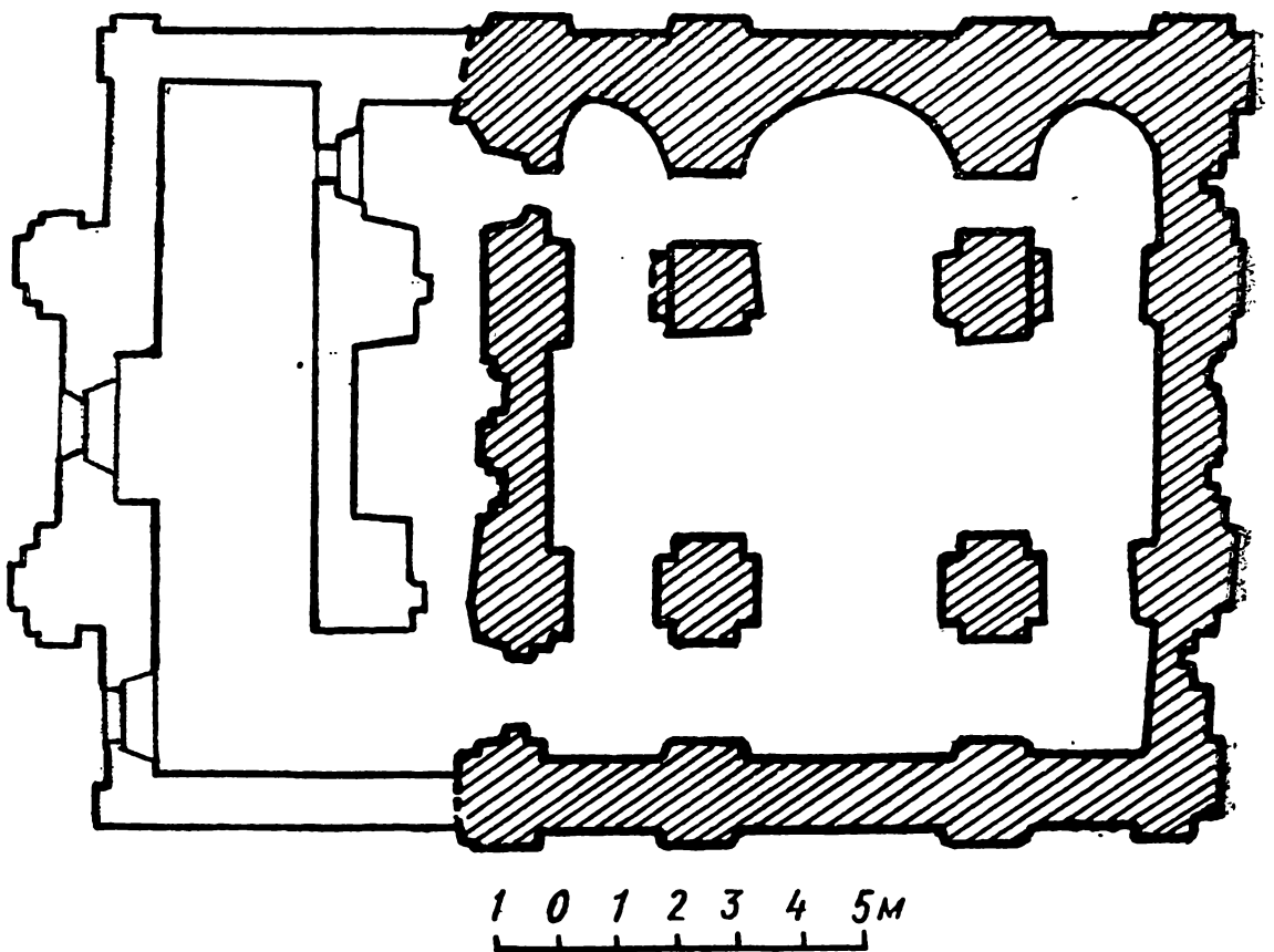
Рис. 15. План Троїцької надбрамної церкви (за обмірами І. В. Моргилевського).
