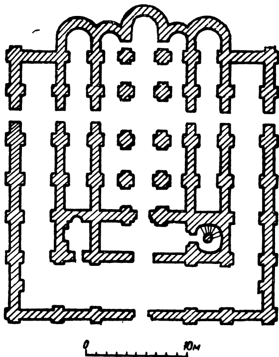
Рис. 38. Храм Кловського монастиря (реконструкція плану).
