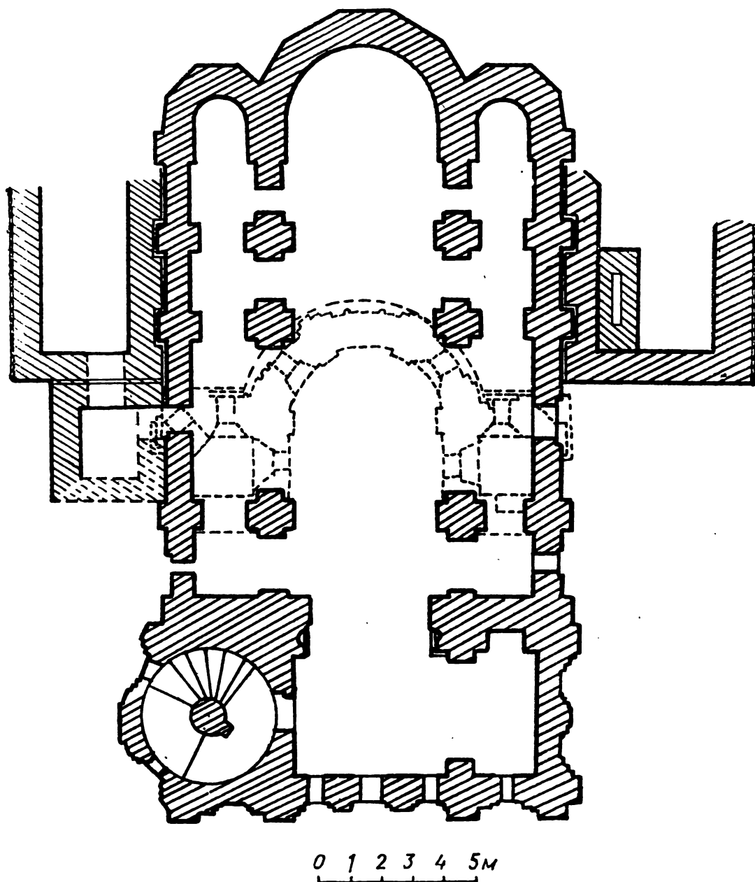
Рис. 26. Михайлівська церква. План першого ярусу (реконструкція М. К. Каргера).
