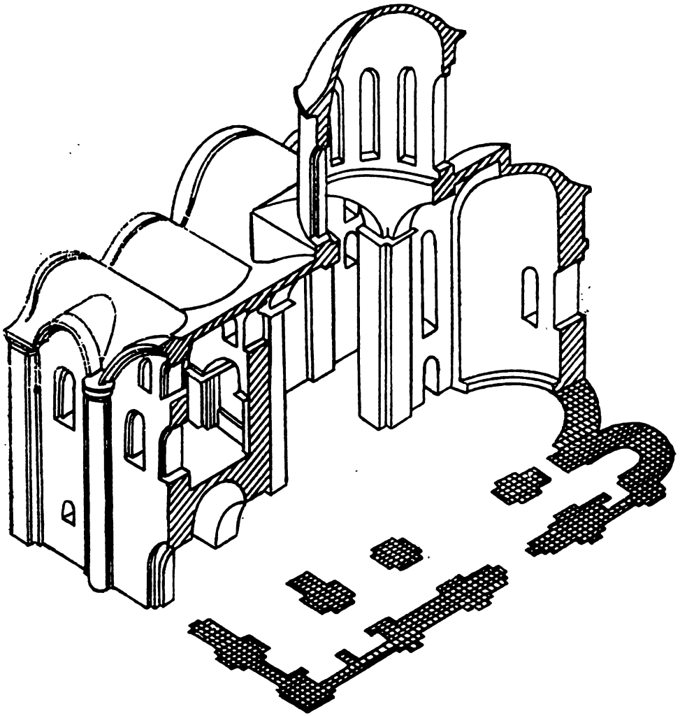
Рис. 42. Церква Кирилівського монастиря (аксонометрія Ю. С. Асєєва).
