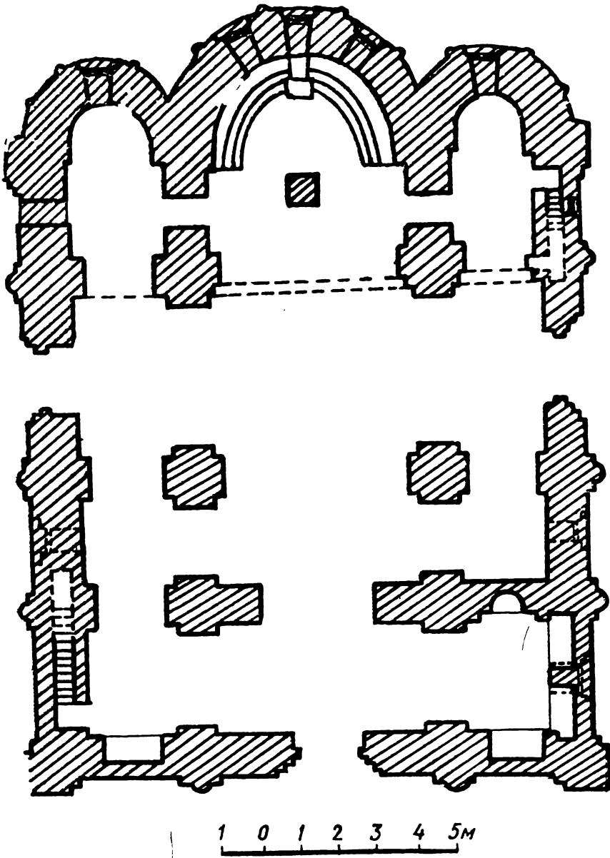
Рис. 41. Кирилівська церква. План першого ярусу.
