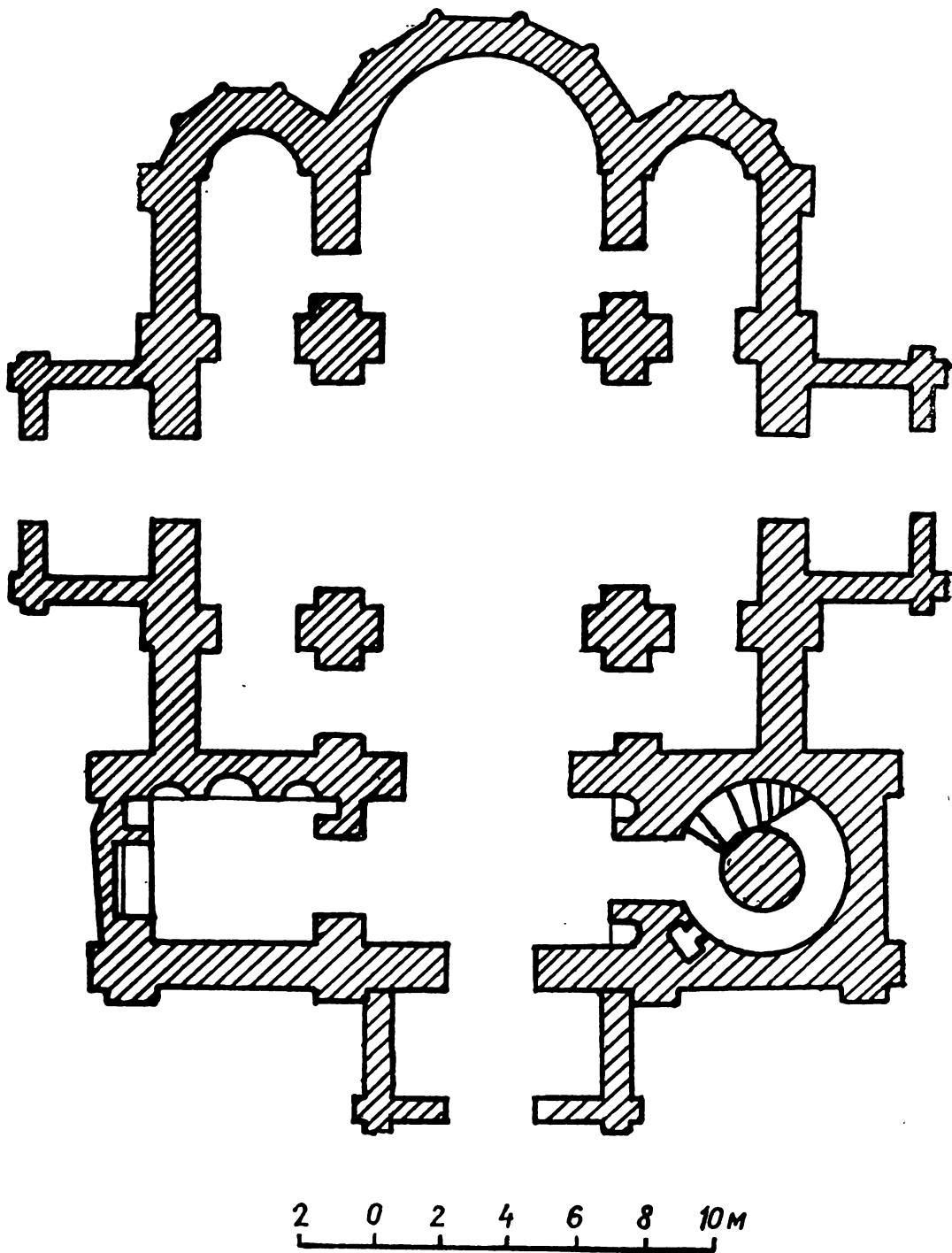
Рис. 5. План церкви Спаса на Берестові (за М. К. Каргером).
