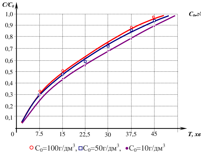
Рис. 8. Ефект очищення води методом цементації в залежності від вихідної концентрації міді
