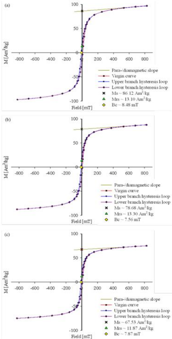
Рис.18.Петля гистерезису зразка ІН28.
