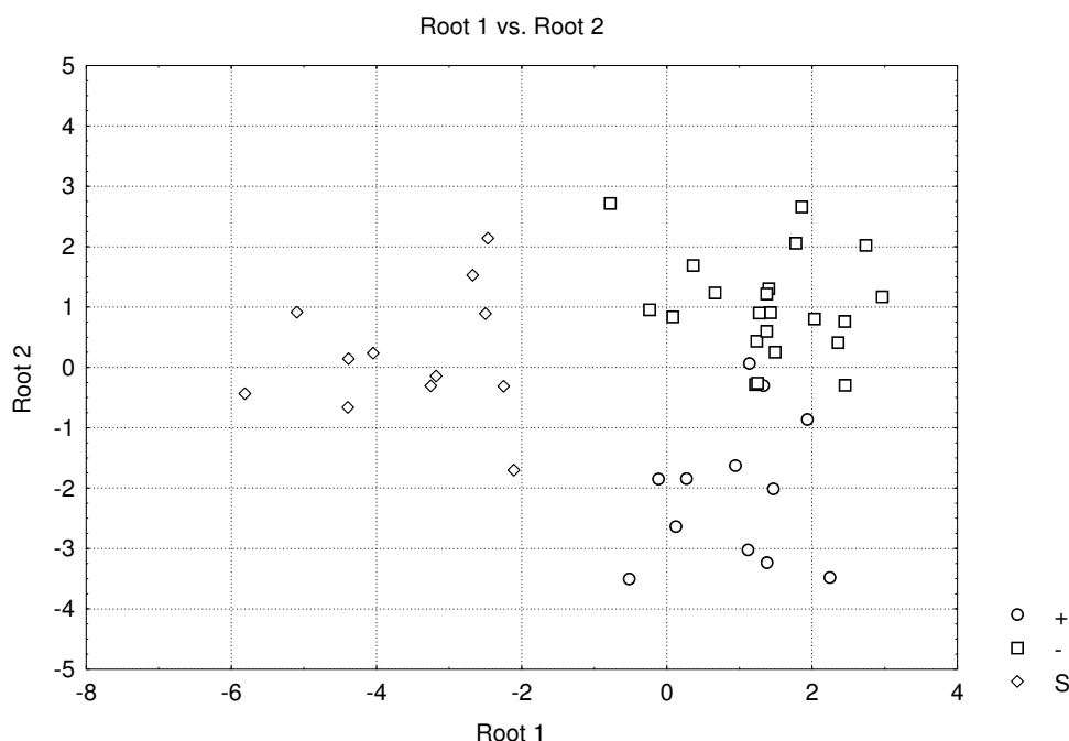
Рис. 5.25. Діаграма розсіювання канонічних значень перших двох радикалів осіб різних типів зв'язків між ICRP та Na,K-ATPase
