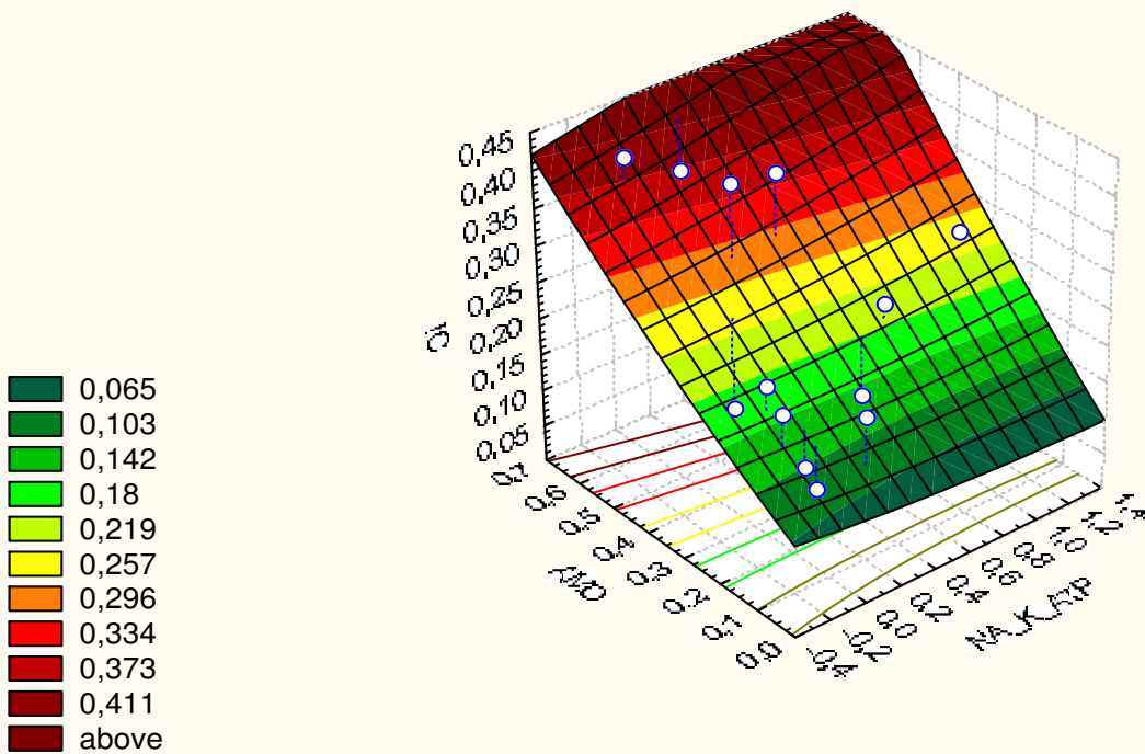
Рис. 5.21. Дигіталісезалежний позитивний інотропний ефект \ln(IC)=0,048-0,028\ln(\text{Na,K-ATP})+0,462\ln(\text{AMo})+0,009\ln(\text{Na,K-ATP})^2+0,138 \ln(\text{Na,K-ATP})*\ln(\text{AMo})+0,142 \ln(\text{AMo})^2
