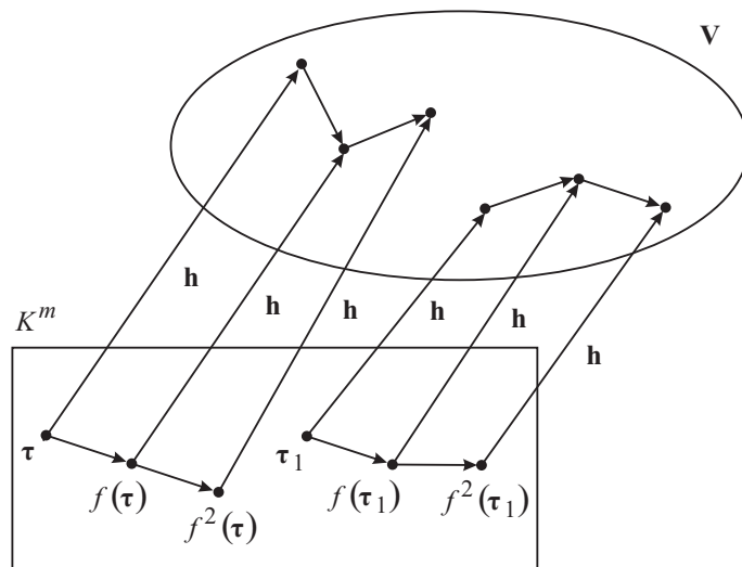
Рис. 6.1. Траектории в многообразии V \in \mathcal{V}_{2,n}(\mathcal{K}) .
