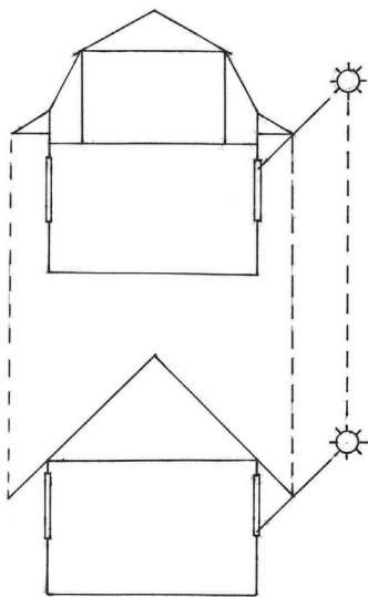
Рис. 15. Порівняння можливостей випуску стріхи в будинку з ломаним дахом і будинку зі звичайним двоскатним дахом
