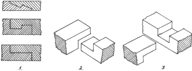
Рис. 7. Види з'єднань підвалин і платів: 1 — повздовжнє; 2 — кутове; 3 — поперечне
