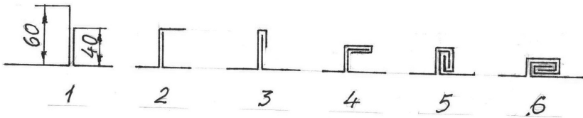
Рис. 18. Подвійний рубець: 1 — згинання листів; 2 — згинання широкої полицьки; 3 — стоячий рубець; 4 — згинання рубця; 5 — подвійний стоячий рубець; 6 — лежачий подвійний рубець
