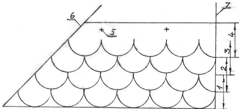
Рис. 19. Послідовність зашивки фронту: 1, 2, 3, 4 – послідовність монтажу смужок; 5 – місця кріплення смужок гвіздками; 6 – дах будівлі; 7 – відкос дверей чи вікна
