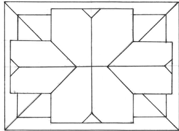
Рис. 11. Схематичне зображення даху зі зламами у трьох площинах і чотирма кімнатами на другому поверсі
