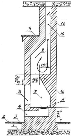
Рис. 21. Камін в розрізі; 1 — фундамент (залізобетонне перекриття); 2 — підлога; 3 — лист заліза; 4 — піддувало; 5 — колосникова решітка; 6 — Вікно каміну; 7 — топка; 8 — димоприймальна камера; 9 — полицка; 10 — димохід; 11 — шибер поворотний; 12 — зуб каміну
