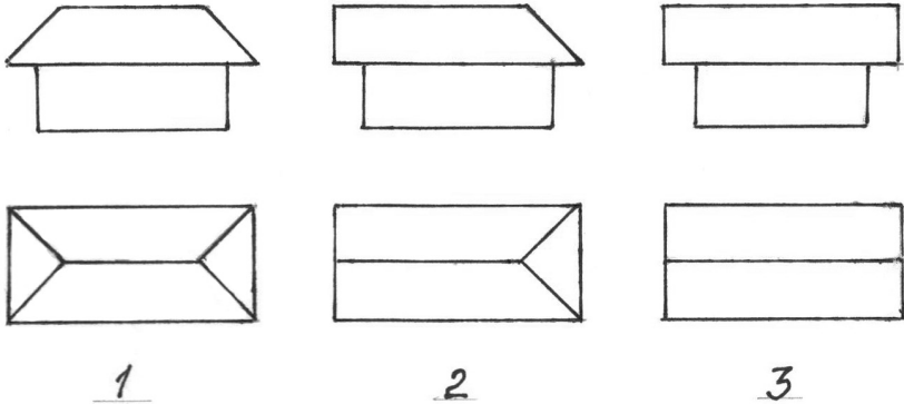
Рис. 10. Схематичне зображення типів дахів: 1 – чотирискатний; 2 – трискатний; 3 – двоскатний
