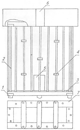
Рис. 31. Конструкція кошниці: 1 – стовпчики; 2 – кілки; 3 – підлога; 4 – бантини; 5 – вікно для виймання кукурудзи; 6 – дверцята для засипання кукурудзи; 7 – підвалини
