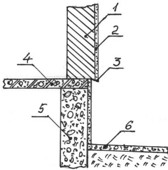
Рис. 26. Кладка стін будинку зі сльозниками: 1 – стіна; 2 – штукатурка; 3 – сльозник; 4 – залізобетонне перекриття; 5 – фундамент; 6 – доріжка
