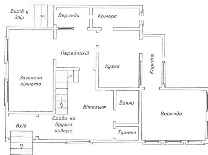
Рис. 24. План першого поверху
