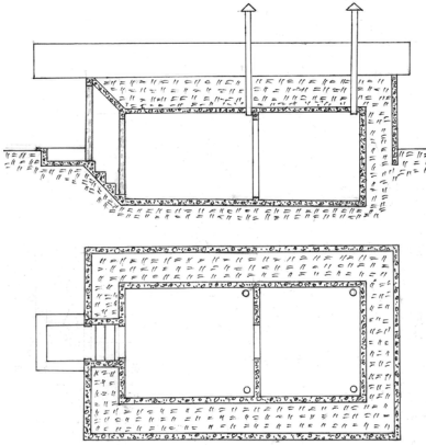
Рис. 29. Пивниця на два відділення з дахом
