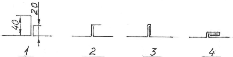
Рис. 17. Одинарний рубець: 1 — згинання листів; 2 — згинання ширшої полицки; 3 — стоячий одинарний рубець; 4 — лежачий одинарний рубець
