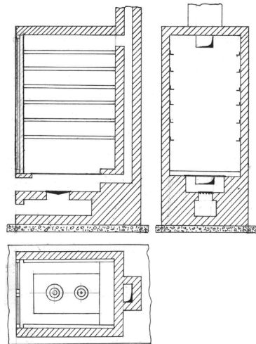
Рис. 30. Сушарка-бужарка
