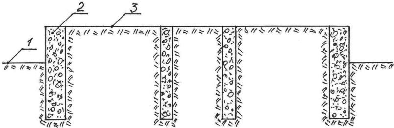
Рис. 5. Розріз фундаменту: 1 — рівень ґрунту будівельного майданчика; 2 — фундамент; 3 — рівень насипного ґрунту
