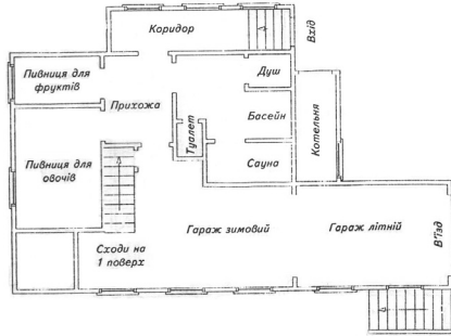
Рис. 23. План підвального поверху
