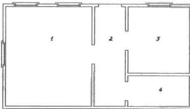
Рис. 3. План хати на дві кімнати: 1 — велика кімната; 2 — хорони (сіни); 3 — мала кімната; 4 — комора
