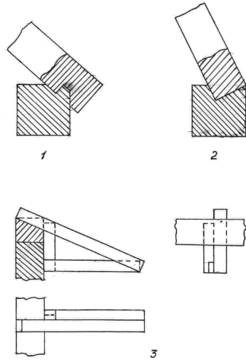
Рис. 14. Закріплення крокв: 1 — на платвах стільця; 2 — на платвах обв'язки; 3 — закріплення крокв стріхи
