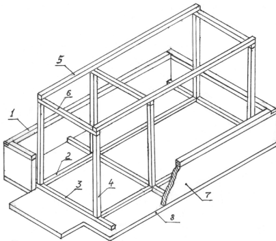
Рис. 12. П-подібний «стілець»: 1 — платва обв'язки; 2 — повздовжня підвалина; 3 — поперечна підвалина; 4 — слупи; 5 — повздовжня платва стільця; 6 — поперечна платва стільця; 7 — стінка; 8 — перекриття з випуском під балкон
