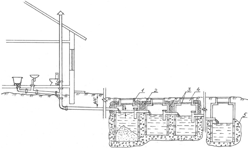
Рис. 27. Обладнання суміщеної каналізації і очистки: 1 — очисна камера; 2 — глиняний замок; 3 — кришка верхня і нижня; 4 — утеплювач (Мінеральна вата, пінопласт, солома); 5 — шутер (щебінь)
