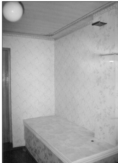
Лежанка з переключенням диму, поштукатурена і обклеєна шпалерами
