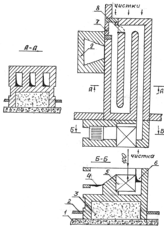
Рис. 22. Плита і триоборотна лежанка: 1 — фундамент (перекриття); 2 — підлога; 3 — наповнювач (пісок, бита цегла); 4 — колосникова решітка; 5 — духовка; 6 — димохід; 7 — димохід лежанки; 8 — шибер поворотний; 9 — камін
