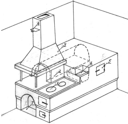
Рис. 20. Традиційна для Покуття конструкція опалювального комплексу: 1 – плита; 2 – піч; 3 – комин; 4 – шибер; 5 – духовка; 6 – котел для підігріву води; 7 – ніша для дров
