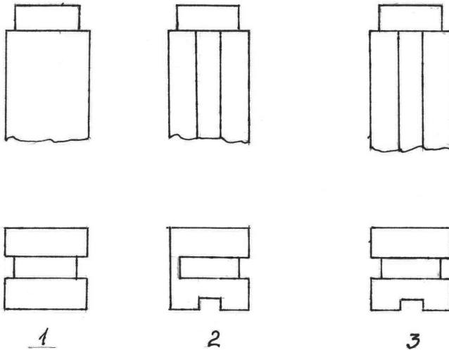
Рис. 8. Види слупів: 1 — стіновий слуп; 2 — кутовий; 3 — з'єднувальний слуп
