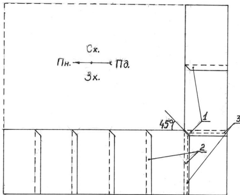
Рис. 16. Схема укладки шиферу: 1 — полоса перекриття горизонтальна; 2 — полоса перекриття вертикальна; 3 — ліній прокладки смужок поролону
