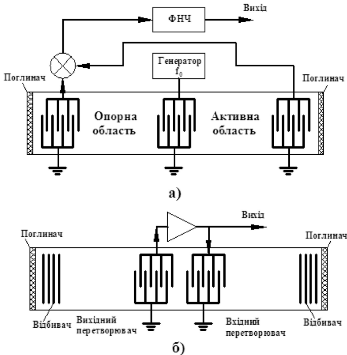
Рис. 1. Типи ПАХ-датчиків:
