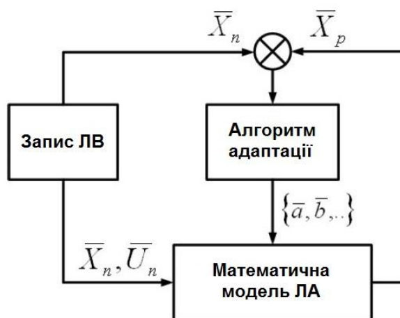
Рис. 2. Блок схема методики ідентифікації аеродинамічних коефіцієнтів на основі синтезу адаптивної системи
