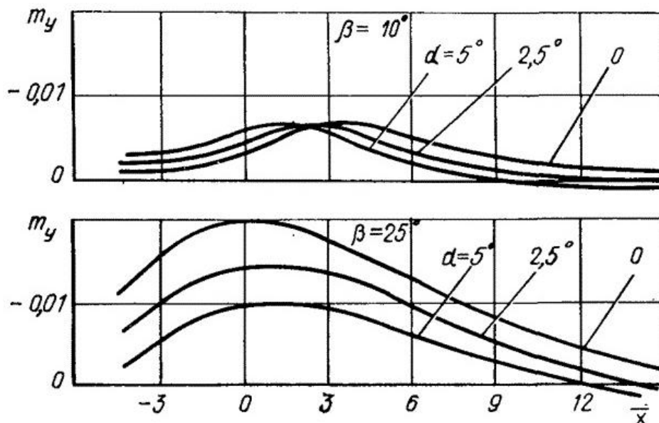
Рис. 1. Залежність аеродинамічного моменту рискання m_y від відносного положення літака вздовж осі трампліна \bar{x}
