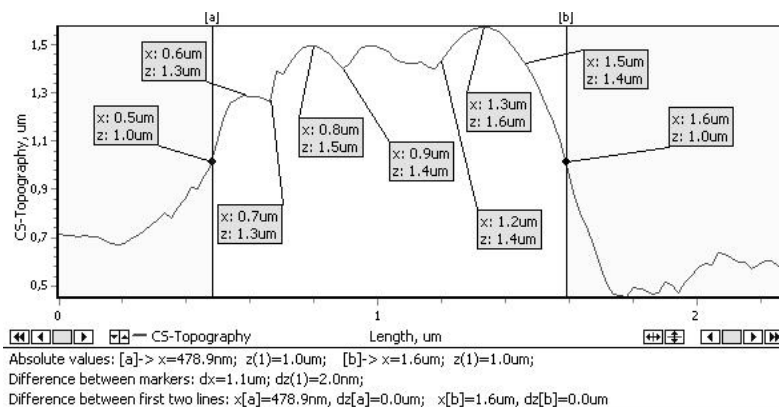
Рисунок 3 – Профіль перетину покриття Fe-Мо-W на підкладці зі Ст.3
