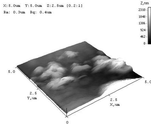
Рисунок 2 – 3-D карта поверхні покриття Fe-Мо-W на підкладці зі Ст.3
