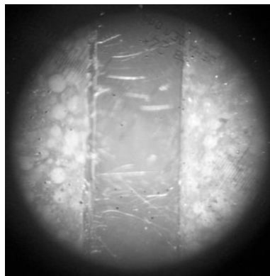
Рисунок 4 – Поперековий переріз покриття Fe-Мо-W на підкладці із Ст.3
