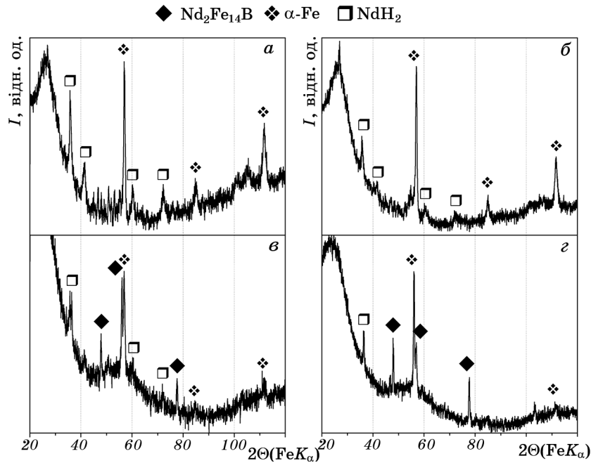
Рис. 3. Дифрактограми стовів \text{Nd}_{16}\text{Fe}_{76}\text{B}_8 ( a , б ) та \text{Nd}_{11,8}\text{Fe}_{82,3}\text{B}_{5,9} ( б , г ) після солід ГД за тиску водню 0,05 МПа при 760°C. Дифрактограми в і г зняли після орієнтування частинок порошку в магнетному полі.
