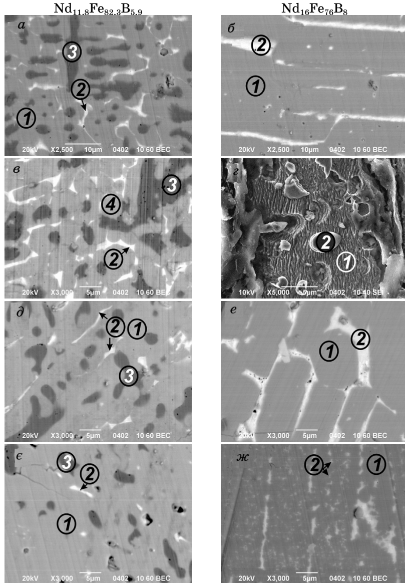
Рис. 5. Мікроструктура стопів: у вихідному стані ( a, б ), після солід ГД ( в, г ) та наступного ДР за температур 770 ( д, е ) і 840°C ( е, ж ); шліф нещавлений: 1 — \text{Nd}_2\text{Fe}_{14}\text{B} , 2 — твердий розчин неодим–залізо, 3 — залізо, 4 — продукти диспропорціонування ( \text{NdH}_{2\pm x} та Fe).
