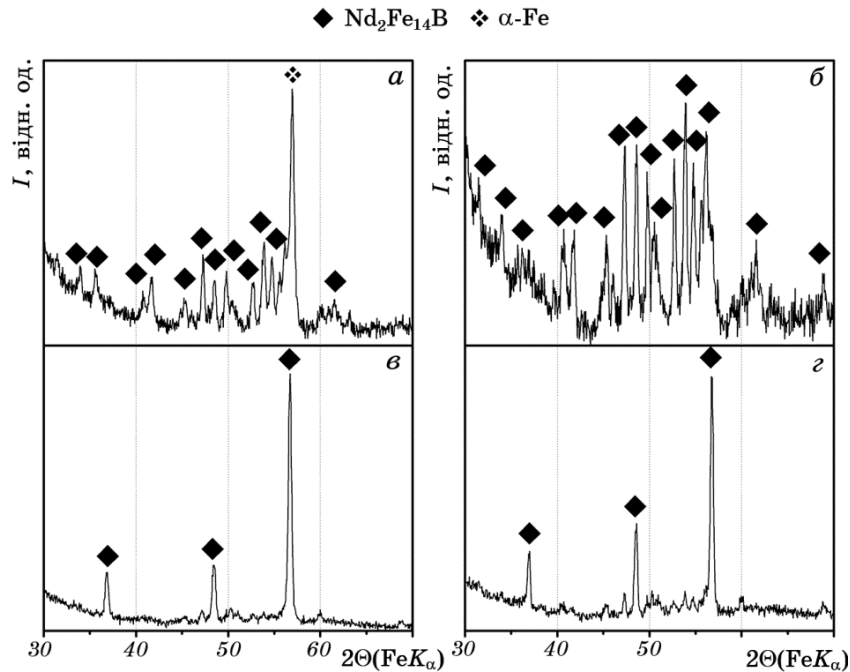
Рис. 4. Дифрактограми стовпів \text{Nd}_{11.8}\text{Fe}_{82.3}\text{B}_{5.9} ( a , c ) та \text{Nd}_{16}\text{Fe}_{76}\text{B}_8 ( b , d ) після десорбування водню з продуктів солід ГДД у вакуум за температури 840^\circ\text{C} . Дифрактограми ( c , d ) зняли після орієнтування частинок порошку в магнетному полі.
