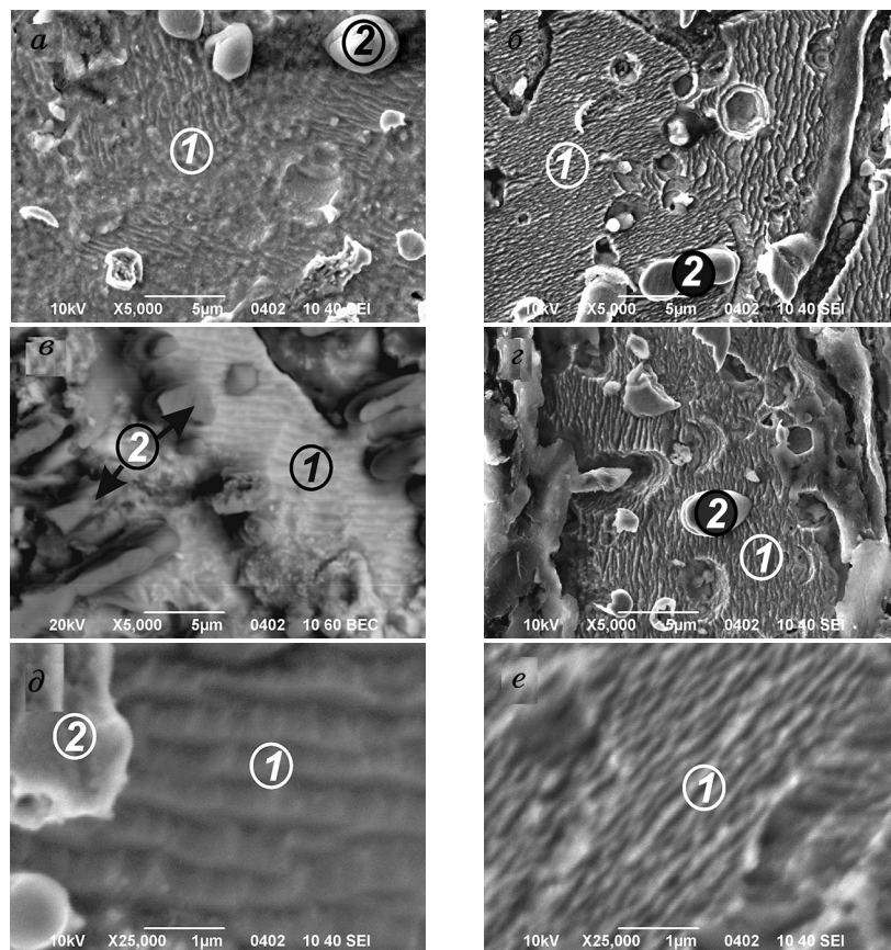
Рис. 6. Мікроструктура ступу Nd 11.8 Fe 82.3 V 5.9 після ДР за температур 770°C (а, в, д) та 840°C (б, г, е); шліф щавлений: 1 — Nd 2 Fe 14 V, 2 — залізо.
