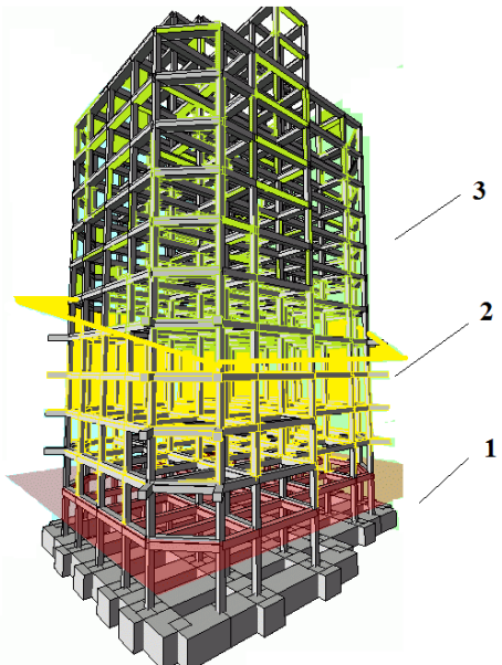
Рис. 1. Розділення висотної будівлі на протипожежні відсіки
