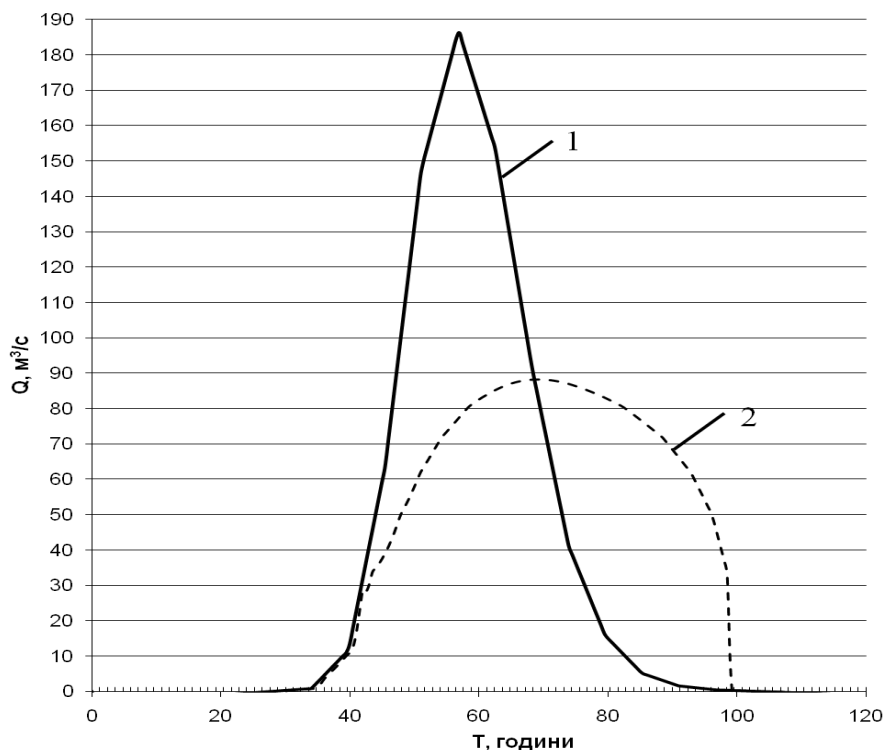
Рис. 2. Трансформація 1% паводкової витрати в сухій гірській ємності:
