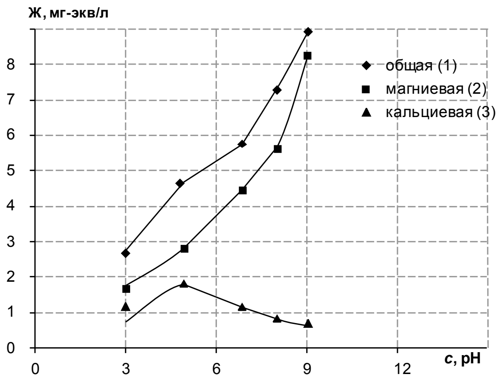
Рис. 3. Зависимость общей, магниевой и кальциевой жесткости от pH воды ( c – pH воды) при скорости фильтрации от 0,5 м/ч до 5 м/ч
