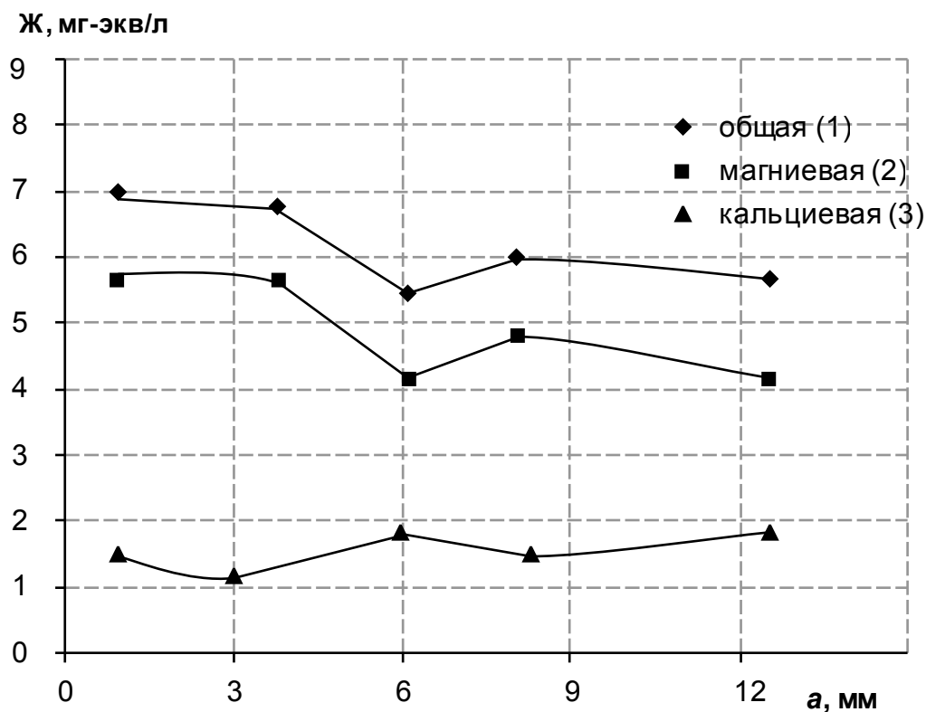
Рис. 1. Зависимость общей, магниевой и кальциевой жесткости от размеров загрузки (a - диаметр, мм) при скорости фильтрования от 0,5 м/ч до 5 м/ч
