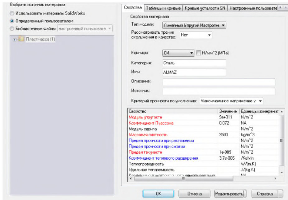
Рисунок 3 – Задание физико-механической свойств зерна марки AC100
