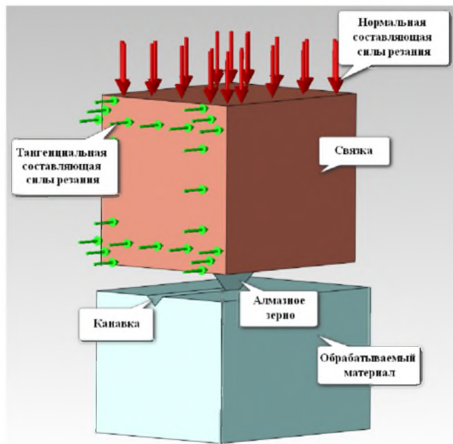
Рисунок 4 – Задание параметров нагружения 3D модели
