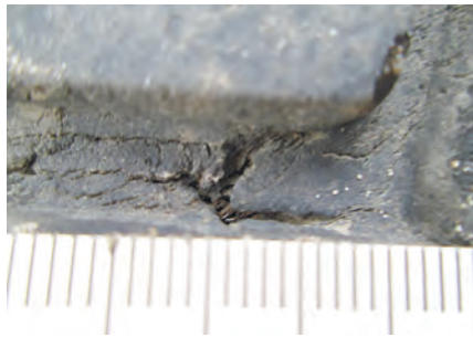
Рис. 7. Пошкодження зовнішнього герметизованого шару протекторної зони шини № 2
