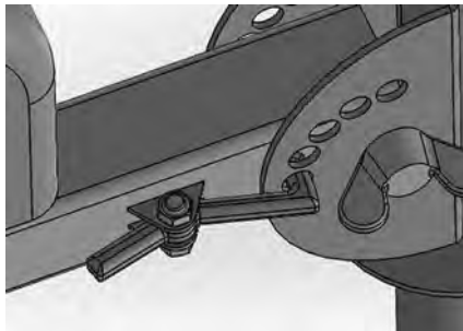
Рис. 4. Детальний вигляд кутового фіксатора
