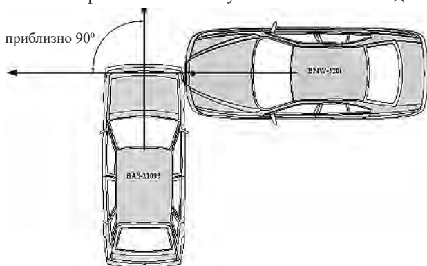
Рис. 2. Взаємне розташування автомобіля BMW-520i та автомобіля ВА3-21093 в момент первинного контакту
