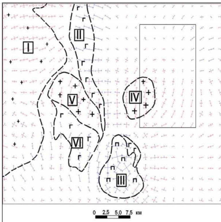
Рис. 3. Поле главных значений тензора чистой деформации района г. Екатеринбург. Массивы: I – Верх-Исетский; II – Шувакишский; III – Уктусский; IV – Шарташский; V – Свердловский; VI – Ширококореченский
