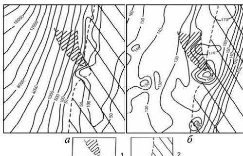
Рис. 2. Распределение удельной энергии деформации (а) – объема, (б) – формы в пределах Естунинского месторождения: 1 – контур месторождения, 2 – область отрицательных значений дилатации
