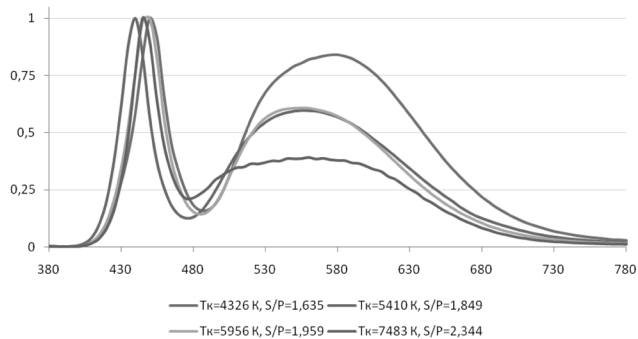
Рис. 2. SPL 2000 Криві спектрального світлорозподілу для джерел світла з різною колірною температурою
