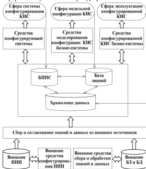
Рис. 5. Обобщенная схема архитектуры КИС бизнес-системы, основанная на концепции конфигураторов
