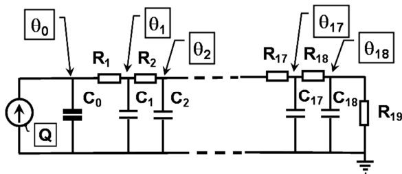
Рисунок 4 - Модель нагрева в виде многоемкостной тепловой цепи
