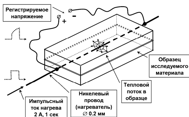
Рисунок 1 – Схема экспериментальной установки для определения удельного теплосопrotивления
