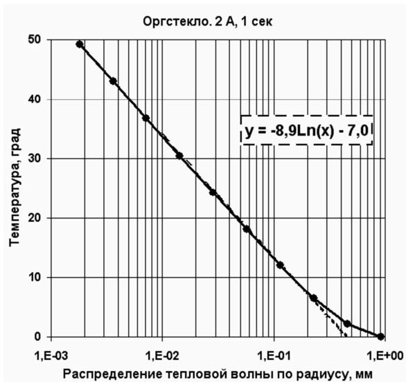
Рисунок 9 - Распределение температуры по радиусу теплового поля через 1 сек от начала прогрева
