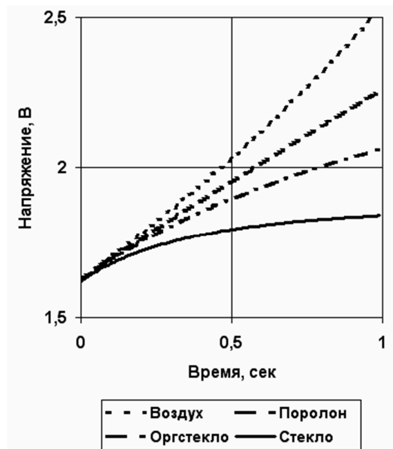
Рисунок 5 - Динамика возрастания электрического напряжения на нагревателе для разных исследуемых материалов. Результаты моделирования
