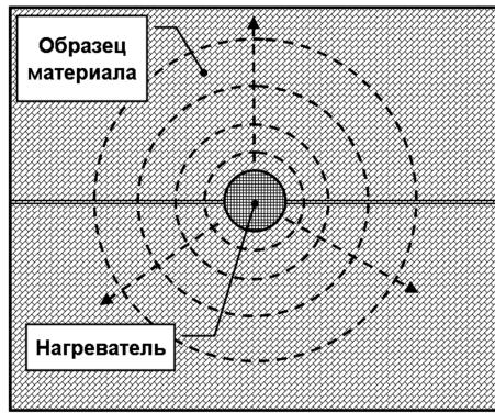
Рисунок 2 - Поперечное сечение теплового поля в случае обволакивающего теплового контакта
