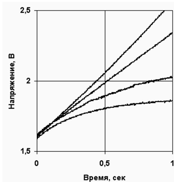
Рисунок 6 – Динамика возрастания электрического напряжения на нагревателе для разных исследуемых материалов. Результаты эксперимента
