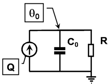
Рисунок 7 – Упрощенная модель нагрева в виде одноемкостной тепловой цепи
