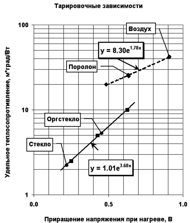
Рисунок 10 – Тарировочные зависимости
