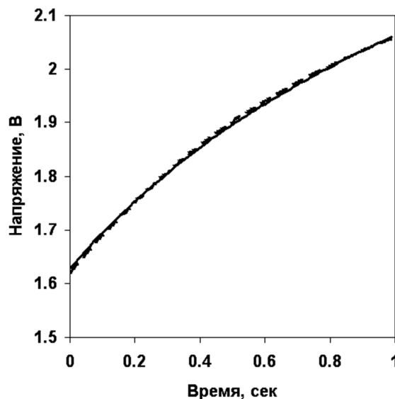
— Многоемкостная модель - - Одноемкостная модель
