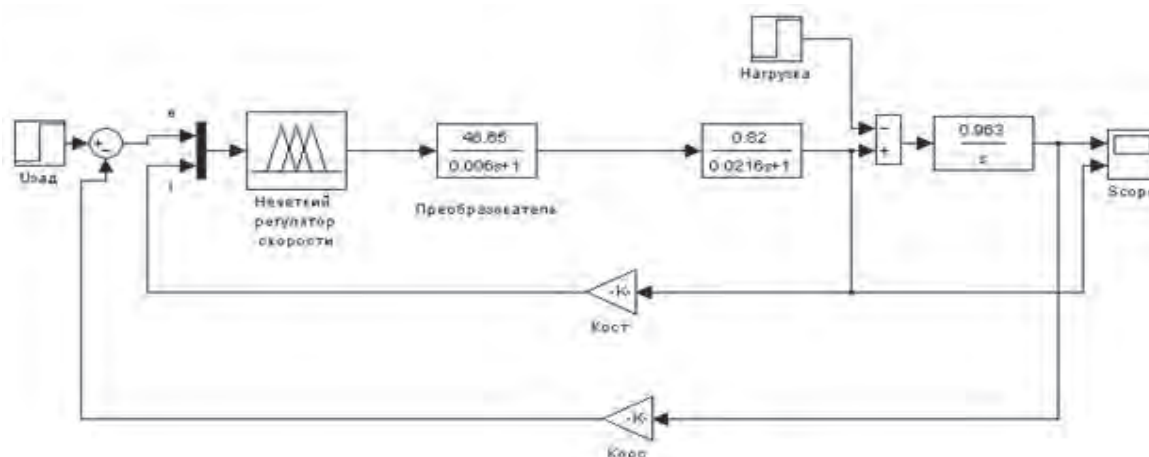
Рис. 3. Модель системи стабілізації швидкості обертання ДПС з нечітким регулятором
