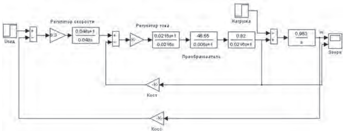
Рис. 1. Повна функціональна схема двоконтурної системи стабілізації в середовищі моделювання Matlab Simulink
