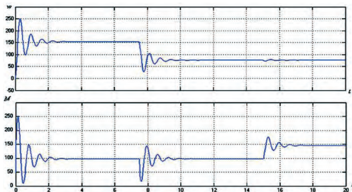
Рис.2. Графік моделювання перехідних процесів класичної системи стабілізації швидкості
