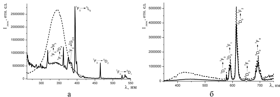
Рис. 3. Спектры возбуждения (а: -\lambda_{\text{лнм}} = 614 нм; ---\lambda_{\text{лнм}} = 420 нм) и люминесценции (б: -\lambda_{\text{возб}} = 280 нм; ---\lambda_{\text{возб}} = 340 нм) Eu-DTPA-APTMS.
