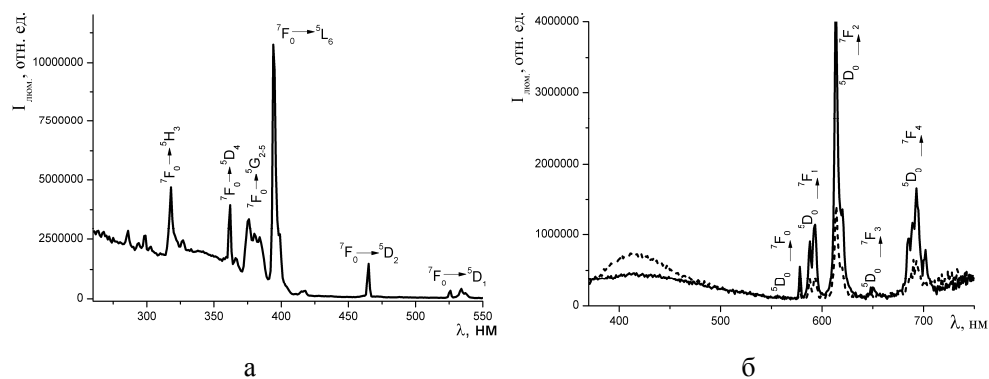
Рис. 6. Спектры возбуждения (а) и люминесценции (б: -\lambda_{\text{возб}} = 280 \text{ нм} ; --- \lambda_{\text{возб}} = 340 \text{ нм} ) Eu-DTPA-APTMS-SiO 2 .
