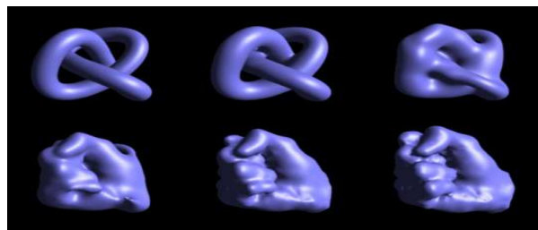
Рис. 4. Анимация – морфинг-метод
