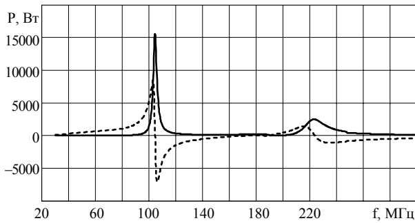
Рис. 3. Комплексная нагрузка антенны:
