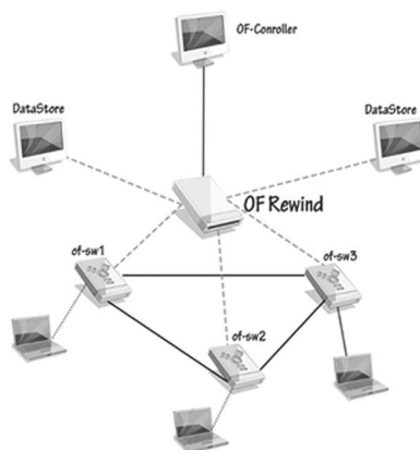
Рис. 2. Системні компоненти OFRewind
