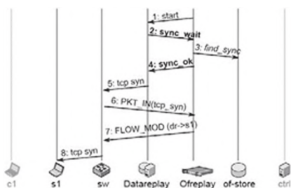
Рис. 3. Приклад використання Ofreplay, коли запит (5: TCP SYN) відправляється із системи зберігання Datareplay від c1
