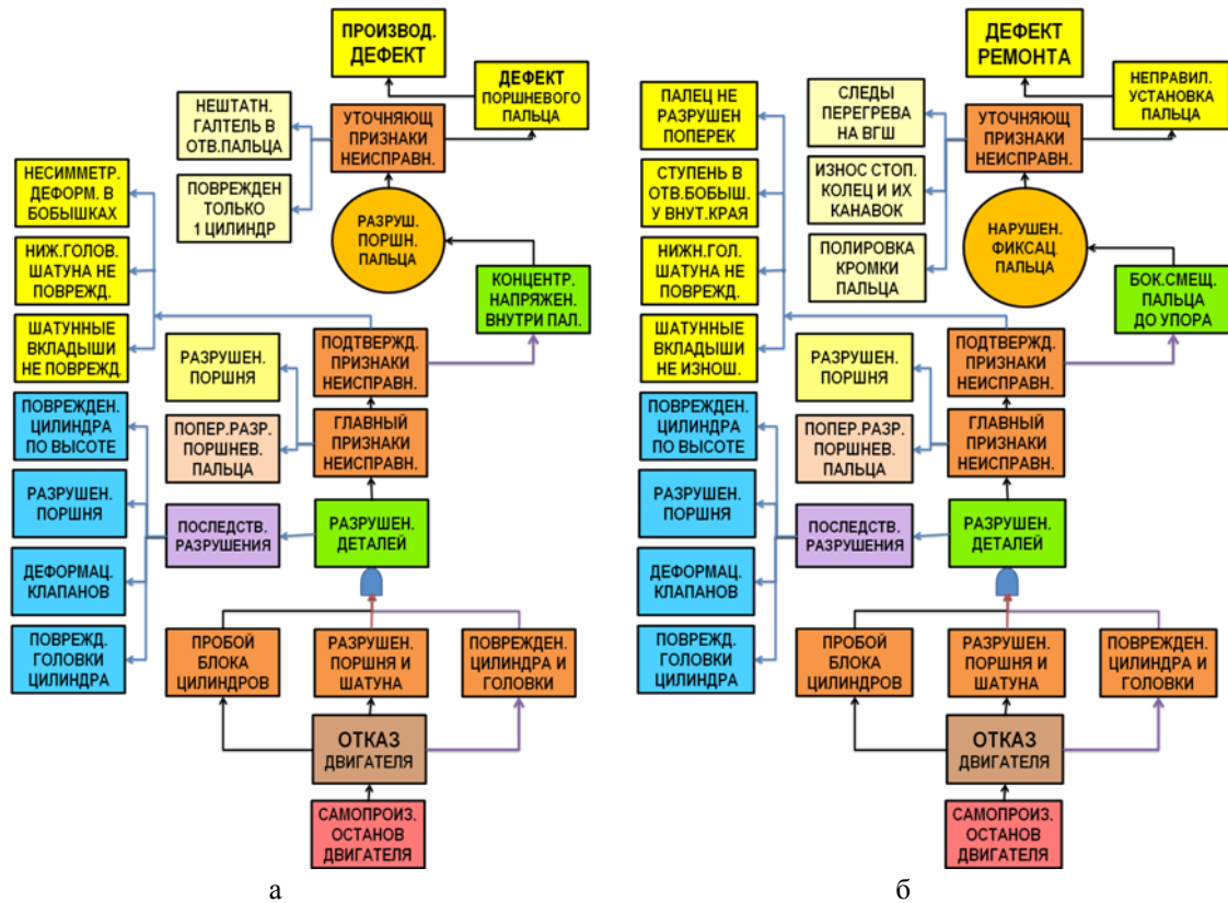
Рис. 6. Общий вид обратного дерева отказа – разрушения поршневого пальца (а) и нарушении его осевой фиксации (б)
