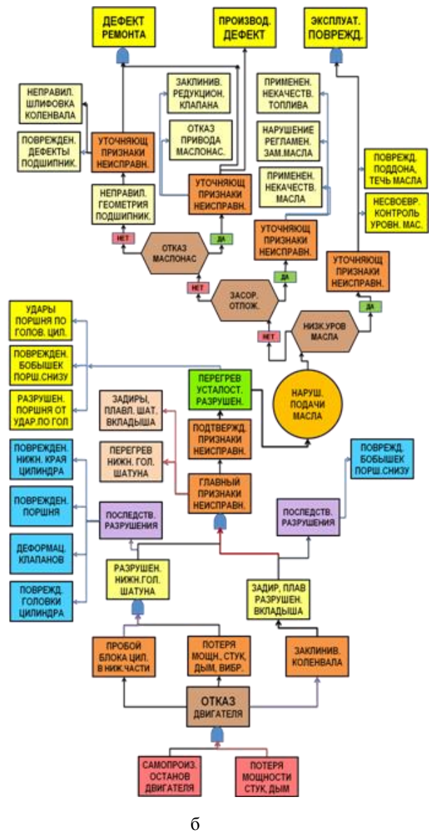
Рис. 5. Общий вид обратного модифицированного дерева отказа двигателя при повреждении и разрушении шатуна после гидроудара (а) и нарушения подачи масла (б)
