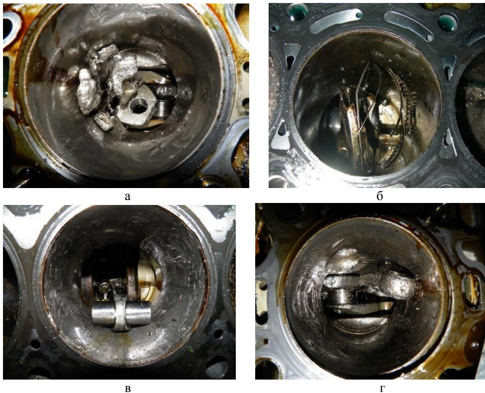
Рис. 7. Последствия тяжелых повреждений двигателей, вызванных отказами с нарушением синхронизации возвратно-поступательного и вращательного движения деталей [4, 16]: а – разрушение поршня и шатуна от недостаточной подачи масла к шатунному подшипнику, б – разрушение шатуна и поршня после гидроудара, в – разрушение поршня после разрушении клапана, г – разрушение поршня после разрушения поршневого пальца
