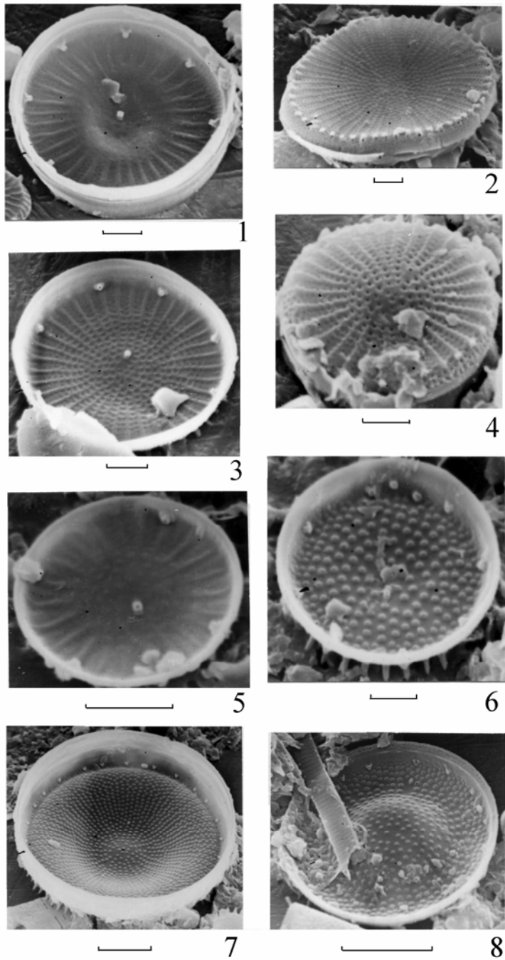
Табл. III. Centrophyceae Камского вдхр.: 1 – Stephanodiscus delicatus ; 2, 3 – S. invisitatus ; 4, 5 – S. makarovae ; 6 – S. minutulus ; 7, 8 – S. neoastraea . 1, 3, 5–8 – створки с внутренней поверхности; 2, 4 – с наружной. Масштаб: 1–6 – 2 мкм; 7, 8 – 10 мкм. СЭМ
