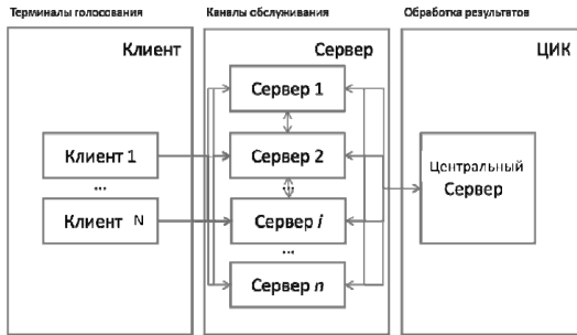
Рис. 3 – Блок-схема СИВ(СИР)
