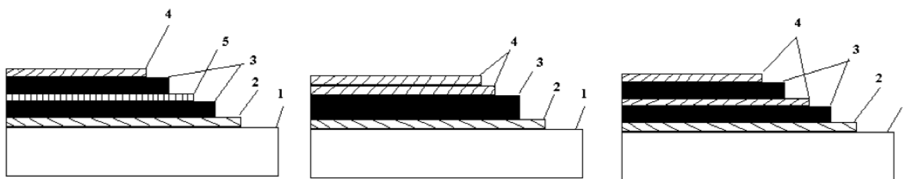
Рис. 2. Конструкції систем покриттів: 1 -сталева основа; 2- грунт "КОНТРАСТ", 3 – покриття бутилкаучуковою герметизуючою мастикою або спеціальним покриттям при потребі; 4 – армувальна сітка згідно з ДСТУ БВ.2.7.-77-98 "Мастики герметизуючі бутилкаучукові" (в співавторстві Баглай А.П., Савенко В.І., Гутніченко Т.П. та ін..) або ДБН В.2.6 – 22 – 2001 Улаштування покриттів із застосуванням сухих будівельних сумішей (в співавторстві Шейніч Л.О., Савенко В.І. та ін..) з відповідним герметиком і фарбуванням 5-фарбування
