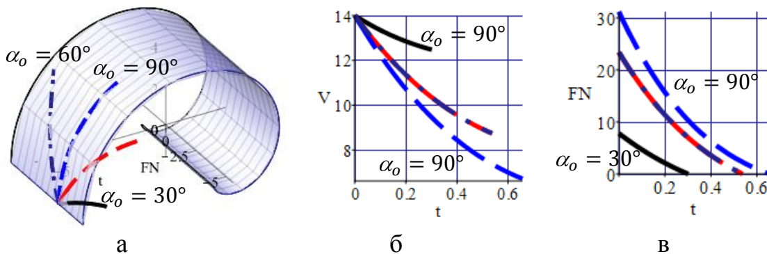
Рис.4. Траєкторії \mathbf{r}(t) та швидкість V(t) частинки по внутрішній поверхні евольвентного циліндра з параметром форми a = 1
