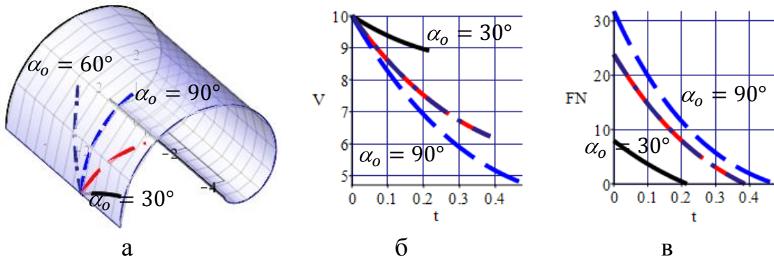
Рис.3. Траєкторії \mathbf{r}(t) , швидкість V(t) та нормальна реакція F_N(t) частинки по поверхні циліндра з початковою швидкістю V_0 = 10\text{м/с}
