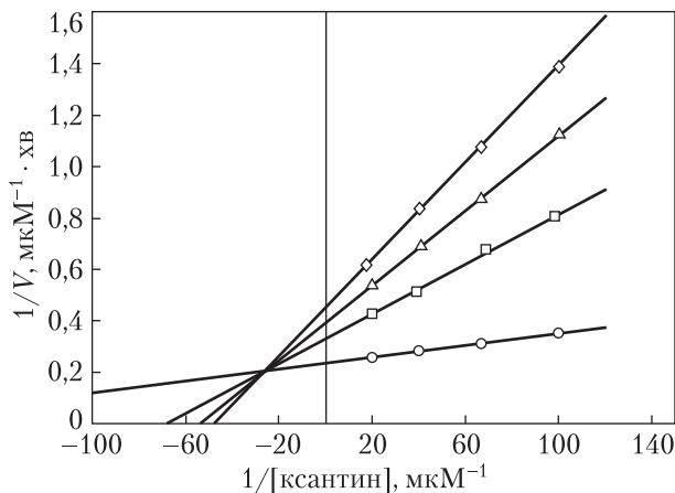
Рис. 1. Графік Лайнуівера–Берка, що описує інгібування активності ксантиноксидази сполукою 3j . Концентрація інгібітора: 0 (○), 2 мкМ (□), 4 мкМ (△) та 6 мкМ (◇)
