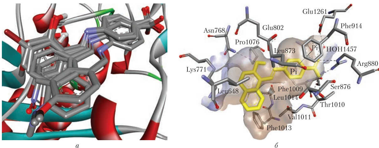
Рис. 2. Суперпозиція азометинових структур 3b , 3d–j в області активного центра ксантиноксидази ( a ) і модель зв'язування сполуки 3j в активному центрі ферменту ( б )
