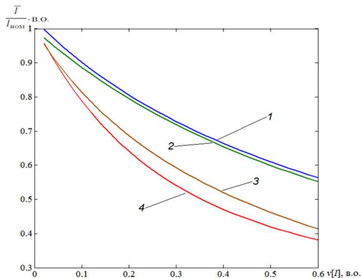
Рис. 2. Характеристики навантажувальної здатності розподільних трансформаторів з охолодженням
