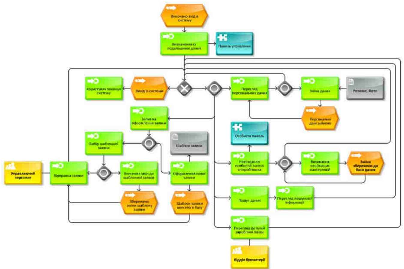
Рис. 3. ЕЕРС-діаграма алгоритму дій користувача в системі інформаційного самообслуговування
