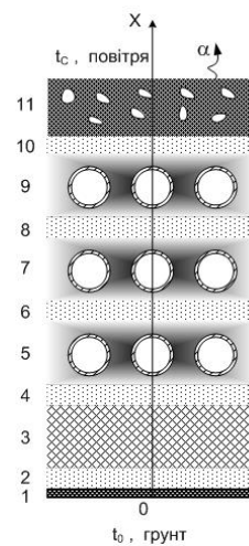
Рисунок 1 – Поперечний переріз багатошарової електрообігрівної підлоги
