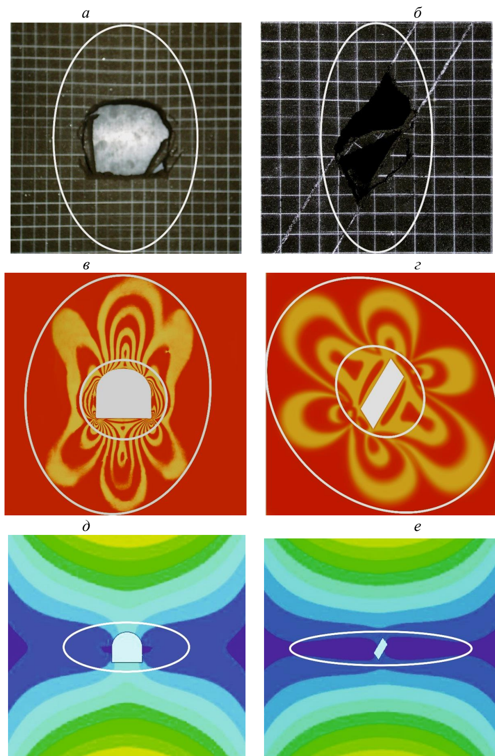
Рис. 1. Результаты выявления энергетических зон при моделировании подготовительных ( а, в, д ) и очистных ( б, г, е ) выработок на эквивалентных ( а, б ), оптико-поляризационных ( в, г ) и электропроводных ( д, е ) материалах: эллиптические линии вокруг выработок – границы зон, где напряжения приближаются к \gamma H
