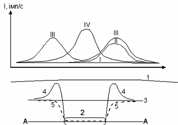
Рис. 1. Модельні криві інтенсивності ПЕМПЗ та перерозподіл гірничого тиску в результаті проведення гірничої розробки 1 – земна поверхня; 2 – підземна гірничая виробка; 3 – вертикальні і горизонтальні напруження вздовж прямої AA до проведення розробки; 4 і 5 – відповідно вертикальні і горизонтальні напруження вздовж прямої AA після проведення розробки; I – відсутні зміни статичного тиску в часі; II – зміна гірничого тиску за рахунок деформації будь-якої стінки камери (наприклад правої на рисунку); III – деформації усіх стінок камери; IV – прогин стелини гірничої камери
