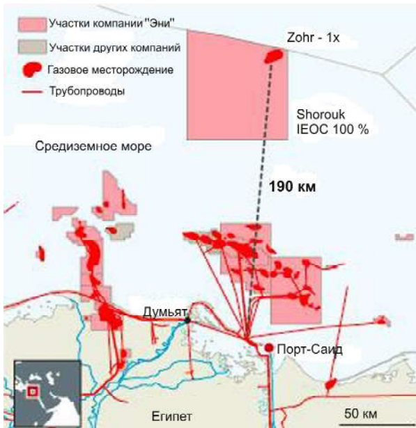
Рис. 3. Положение структуры (месторождения) Zohr в пределах лицензионного блока 9 [15]
