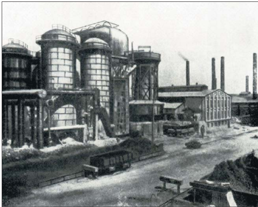
Доменна піч Дніпровського заводу Південно-Російського Дніпровського металургійного товариства. 1896
