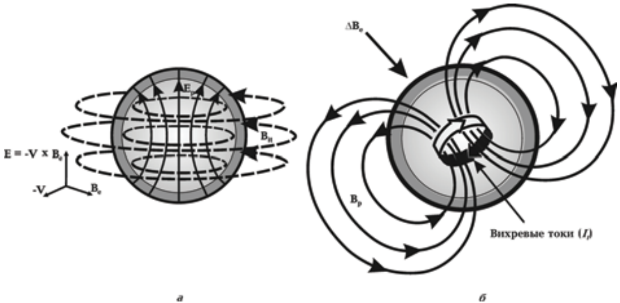
Рис. 4. Торoidalное магнитное поле токов под действием электрического поля -V \times B_s , возникающего в результате движения Луны относительно магнитного поля B_s набегающего солнечного ветра (кондуктивная мода) (а) и полоидальное поле B_p , индуцированное изменениями внешнего магнитного поля \Delta B_s (вихревая мода) (б). Поля даны в предположении, что Луна со всех сторон окружена непроводящей средой.
