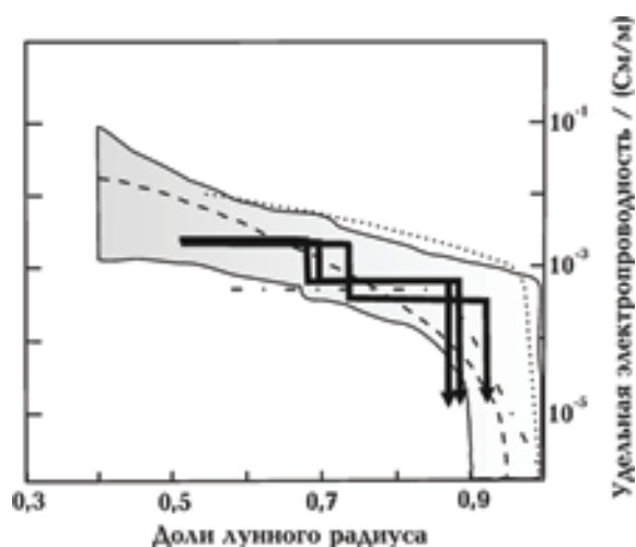
Рис. 9. Модели электропроводности Луны по данным работы [Sonett, 1977].
