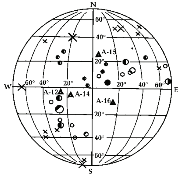
Рис. 1. Карта эпицентров лунотрясений. Кружки — приливные, крестики — тектонические, малый кружок — число лунотрясений менее 5 % от общего, средний — менее 10 %, большой — более 20 %, полый кружок — глубина не определена, залитый на четверть — глубина 500—600 км, залитый наполовину — 600—700 км, залитый полностью — глубина 700—900 км. Треугольниками с соответствующими номерами показаны сейсмические станции "Аполлонов".
