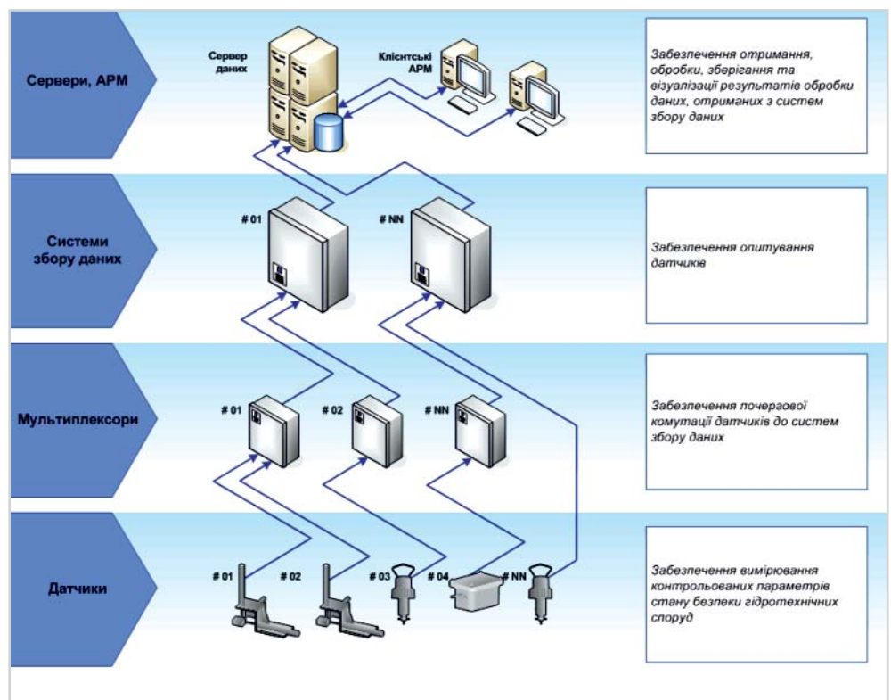
Рис. 4. Принципиальная схема технического оснащения АСК Днестровской ГАЭС.
