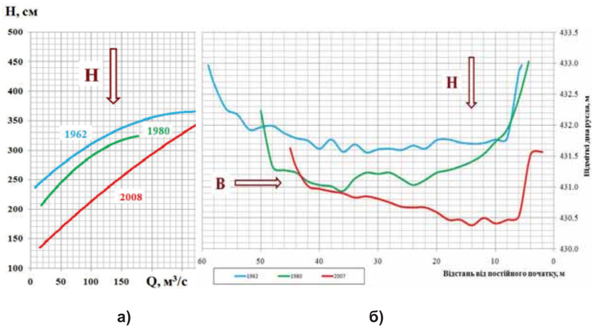
а) б) Рис. 2. Оцінка вертикальних руслових деформацій для ділянки Тиси в м. Рахів на основі: а) кривих витрат води; б) зівставленні різночасових поперечних перерізів русла
