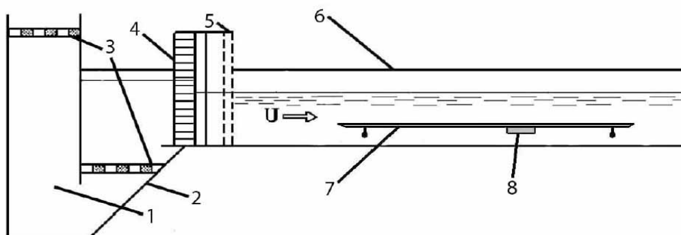
Рис. 2. Схема експериментальної установки: 1 – заспокійлива камера; 2 – конфузор; 3 – решітки; 4 – хонейкомб; 5 – сітки однорідної турбулізації потоку; 6 – гідродинамічний лоток; 7 – пластина; 8 – траншея
