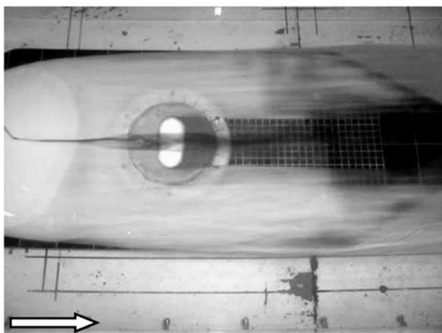
Рис. 5. Візуалізація структури прилежового шару над обтічною пластинною та течії всередині овальної траншеї
