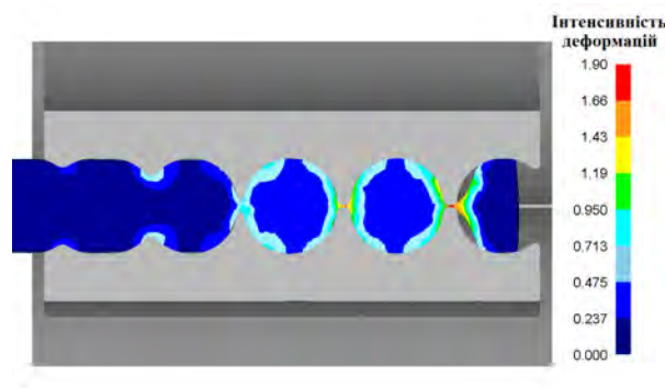
Рис. 11. Розподіл інтенсивності деформацій в поздовжньому розрізі заготовки
