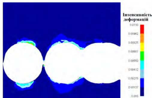
Рис. 13. Розподіли інтенсивності деформацій в поздовжньому розрізі частин валків 2 і 3 в процесі прокатки шариків
