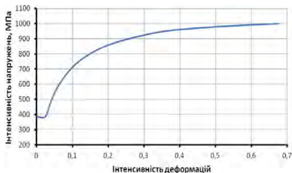
Рис. 9. Крива зміцнення сталі 3Х-15
