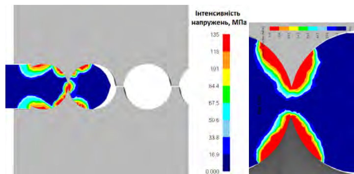
Рис. 6. Розподіл інтенсивності напружень в поздовжньому розрізі заготовки (а) та осередок деформації в заготовці (б)
