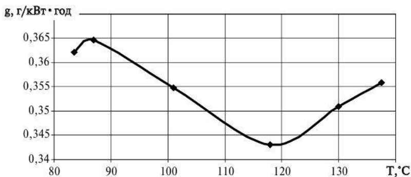
Рис.2. Залежність питомої витрати пального двигуном Д-65Н від температури біопалива під час вприскування в циліндр двигуна за 70% навантаження
