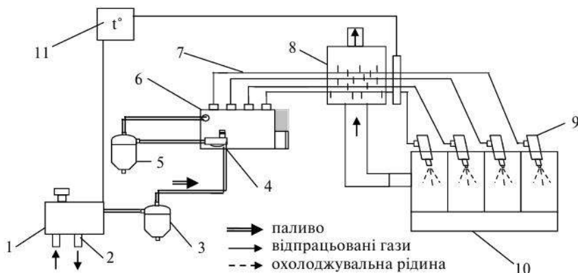
Рис. 1. Схема системи двохступеневого підігріву палива для автотракторних двигунів:
