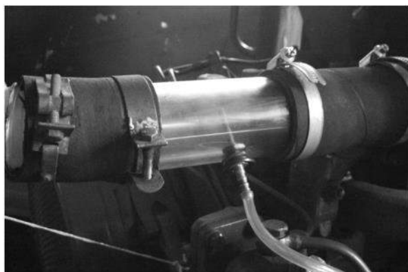
Рис. 3. Подача біоетанолу у повітряний колектор дизельного двигуна Д-21А
