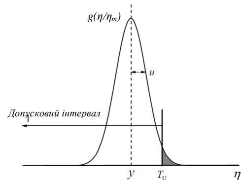
Рис. 2. Поле допуску з однією верхньою границею T_U
