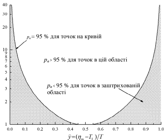
Рис. 3. Діаграма, що показує, за яких співвідношень c_m та \tilde{y} значення ймовірності відповідності p_v залишається сталим і дорівнює 95 %
