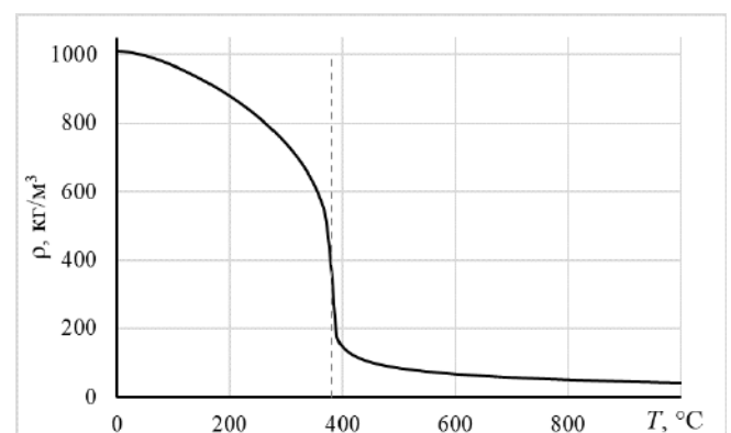
Рис. 1. Температурная зависимость плотности воды при давлении P = 24 МПа
