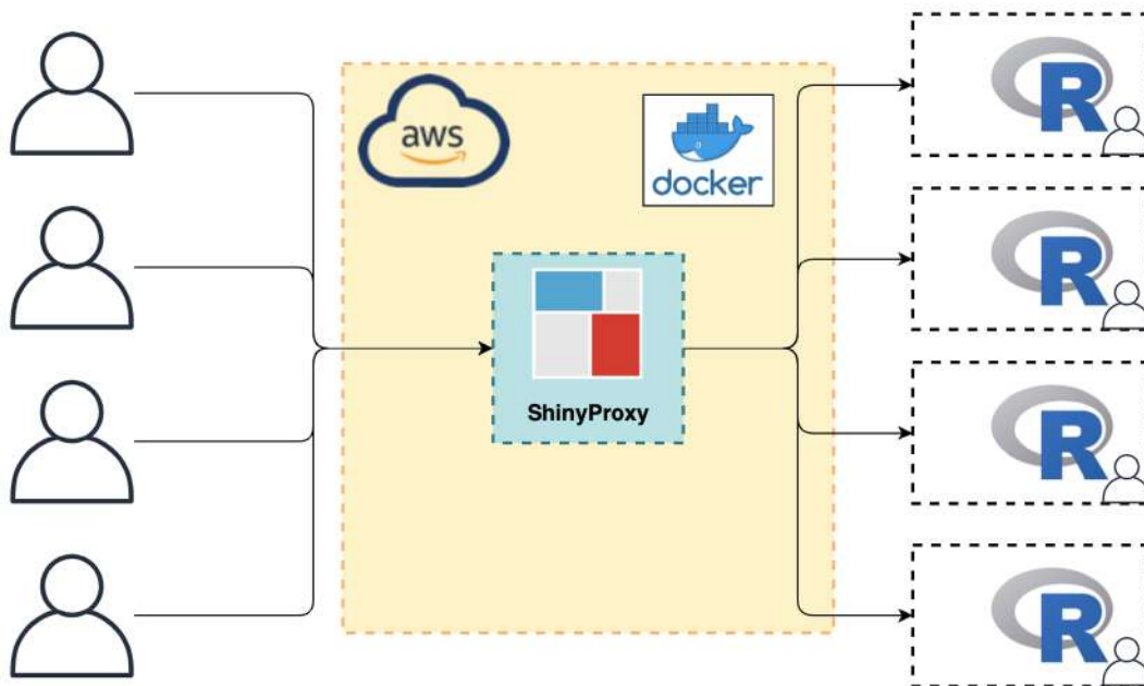
Рис. 2. Архітектура хмарного сервісу
