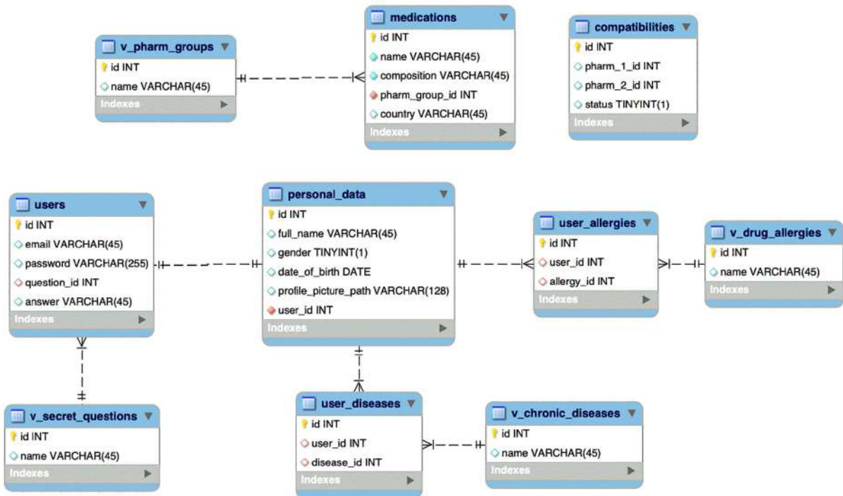
Рис. 1. Діаграма сутність-зв'язок
