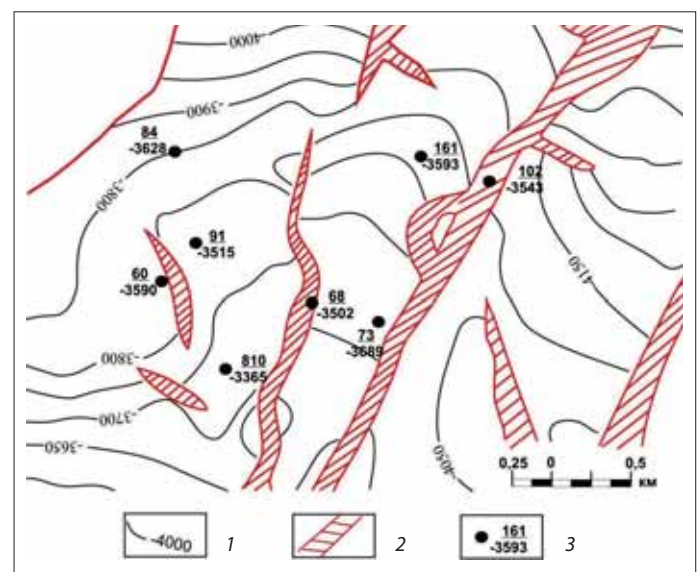
1. Нафтове родовище Білий Тигр – північне склепіння. Структурна карта по покривлі горизонту АФ–СГ. Мірло 1:25000: 1 – ізогіпси покривлі горизонту; 2 – тектонічні порушення; 3 – пробурені свердловини
