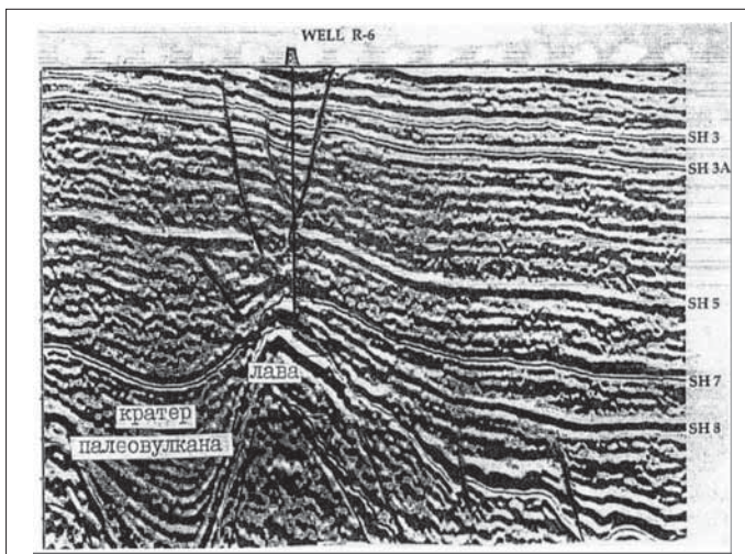
Рис. 2. Нафтове родовище Дракон. Фрагмент сейсмічного розрізу за с. п. DR 93-800
