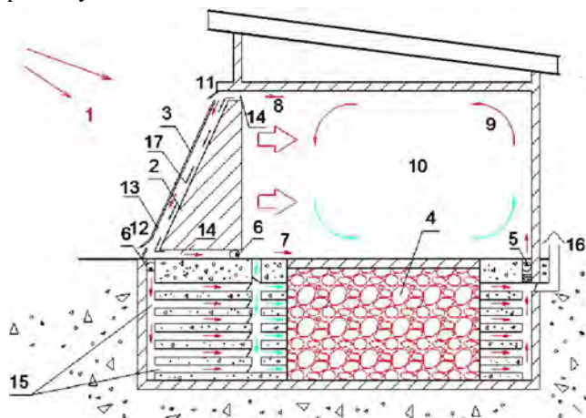
Рис. 1. Схема пасивної системи сонячного обігріву: 1) Сонце; 2) стіна Тромбе-Мішеля; 3) подвійне скління; 4) щебеневий акумулятор; 5, 6) вентилятори; 7) вхідний потік повітря; 8) вихідний потік повітря; 9) потік повітря, нагрітий в акумуляторі; 10) приміщення, що нагрівається; 11, 12) шибери у склінні; 13) проміжок між склінням; 14) циркуляційні канали у стінці Тромбе-Мішеля; 15) канали подавання повітря в тепловий акумулятор; 16) канал відведення повітря; 17) штора
