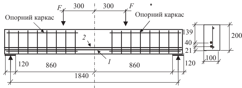
Рис. 1. Конструктивна схема армування дослідних балок Б – 1,2,3: 1, 2 – поздовжні робочі стержні діаметром 12 мм класу A500С
