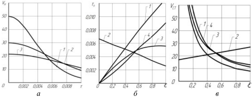
Рис. 2. Залежності нестационарної швидкості росту (а), порогового часу (б) та стаціонарної швидкості росту (в) колонії однофазних зерен при наявності «рухомих» вкраплень. Для кривих v_n(\tau) : 1 - \varepsilon_1=\varepsilon=0,30 ; 2 - \varepsilon_1=\varepsilon=0,5 ; 3 - \varepsilon_1=\varepsilon=0,7 . Для кривих \tau_{II}(\varepsilon) та v_{ст}(\varepsilon) : 1 - \varepsilon_1=\varepsilon ; \varepsilon_2=0 ; 2 - \varepsilon_1=0,5 ; \varepsilon_2=\varepsilon ; 3 - \varepsilon_1=\varepsilon_2=\varepsilon ; 4 - \varepsilon_1=\varepsilon ; \varepsilon_2=0,5 . При розрахунках приймали, що \gamma=3 , L=2 , P=6 , A^*=1 (все в умовних одиницях, що не порушує співвідношень розмірностей)
